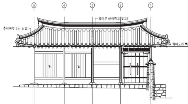
■ 배면도
