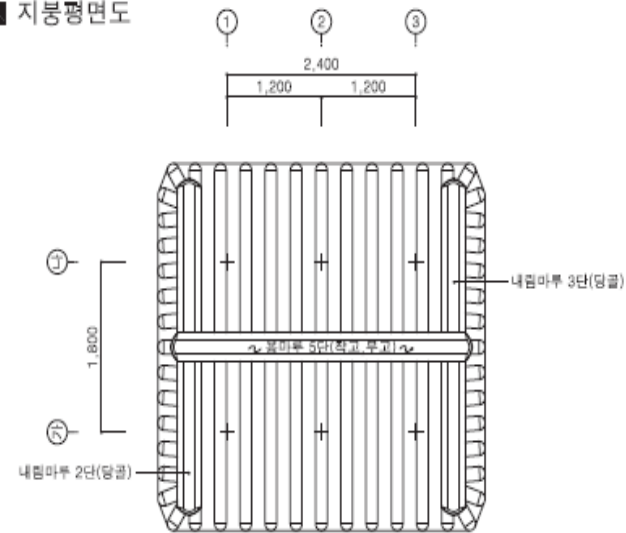
■ 지붕평면도
