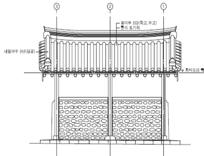
■ 배면도
