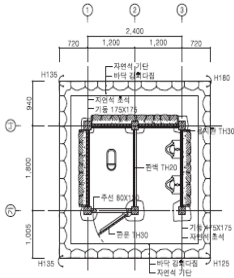
■ 평면도
