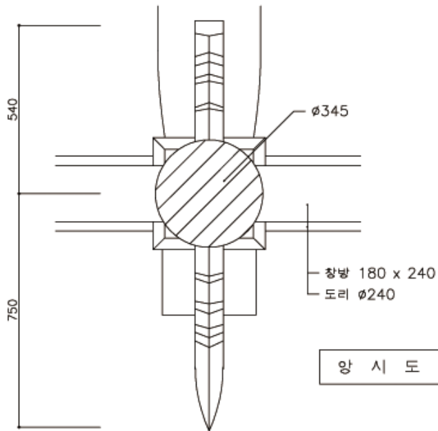
익공 상세도
