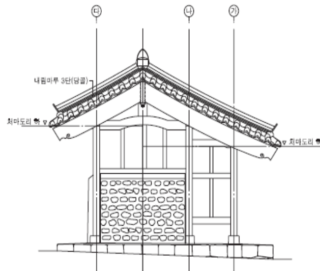
■ 배면도
