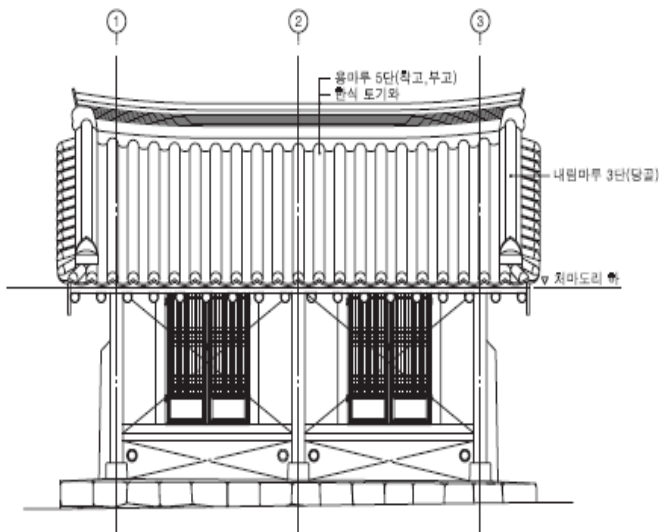
■ 우측면도
