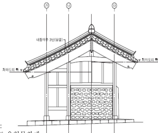
■ 우측면도
